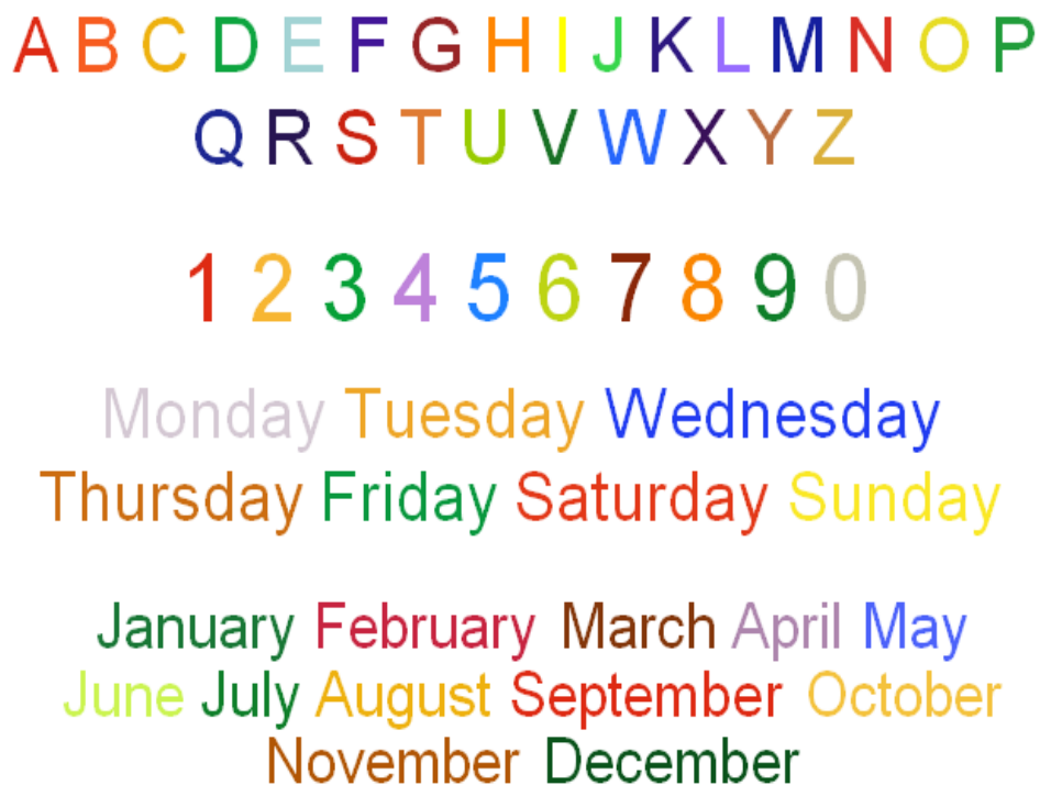
Slika 4. Grafem-boja vrsta sinestezije
