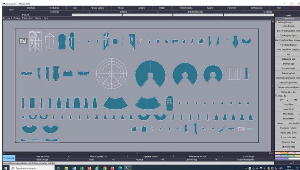
Slika 31: Prikaz krojnih dijelova sa šavnim dodatcima i referentnom osi
