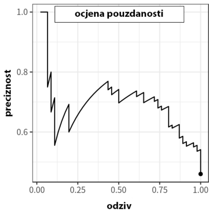
Slika 5 Krivulja preciznost-odziv [8]
