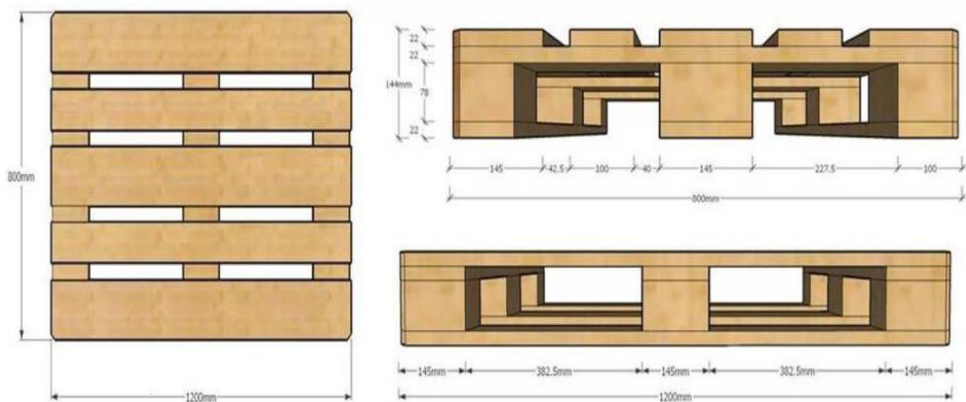
Prilog 1. Dimenzije EPAL Euro palete [14]
