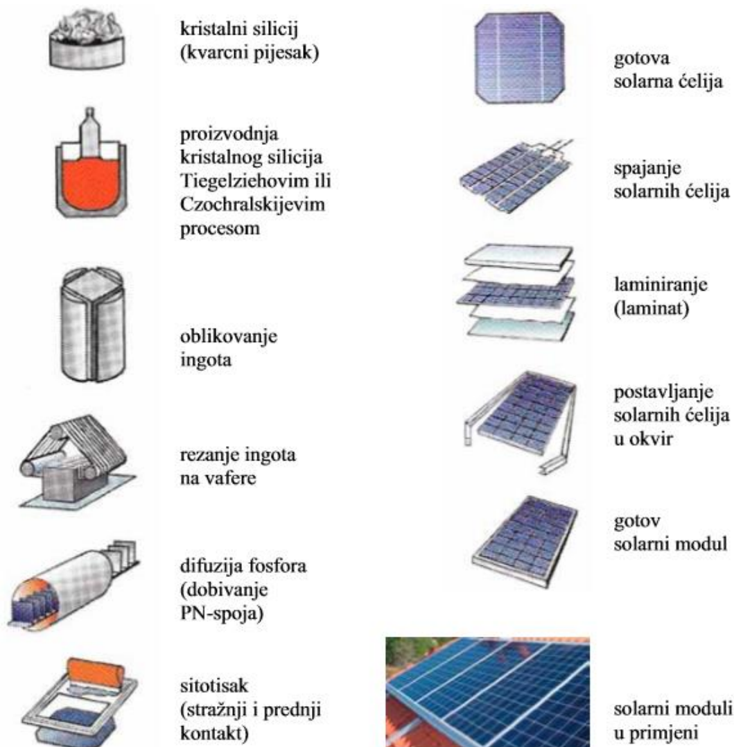
Slika 3.5. Postupak proizvodnje solarnih ćelija i solarnog modula [8]
