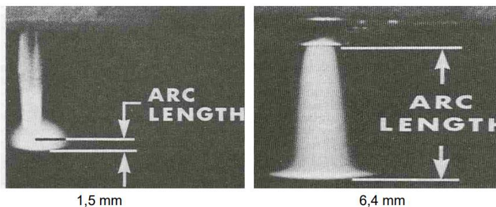
Slika 8.1.5. Usporedba duljine električnog luka (10 A).[43]
