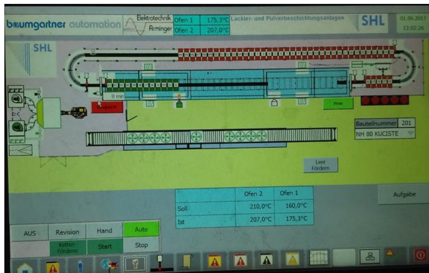
Slika 2.11 Zaslona upravljačke jedinice peći [13]
