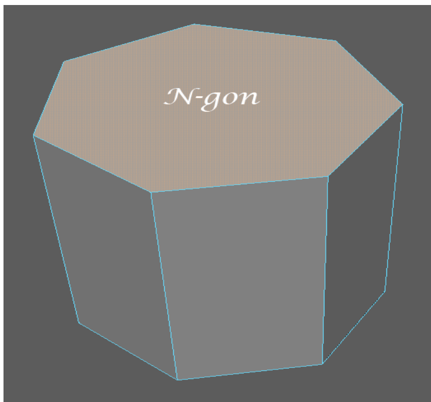
Slika 1-17: Prikaz n-gona
