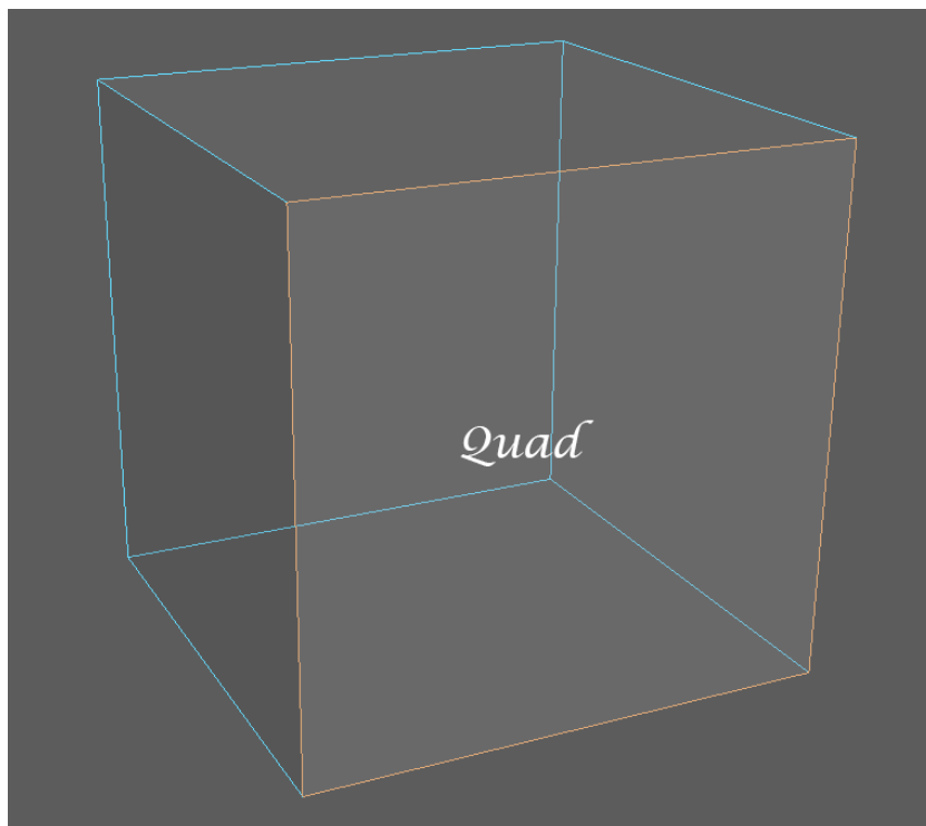
Slika 1-16: Prikaz quadranglea
