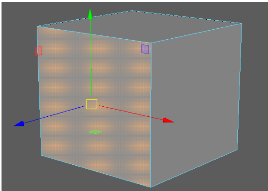
Slika 1-12: Prikaz lica
