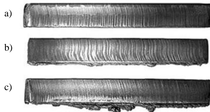
Slika 24. Ovisnost kvalitete rezanja o brzini: a) pogodna brzina rezanja, b) prevelika brzina rezanja, c) premala brzina rezanja
