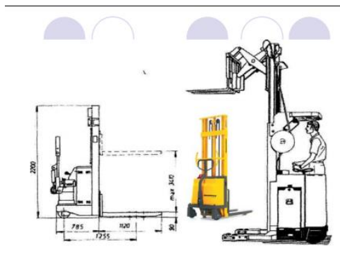
Slika 2.9.: Motorno-ručni viličar [3]
