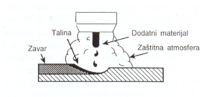
Slika 11. Prikaz zaštitne atmosfere plina prilikom zavarivanja [17]
