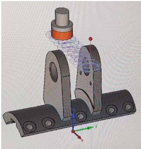
Slika 54. Simulacija glodanja na mjeru 64 mm s glodalom \phi 50 mm [28]
