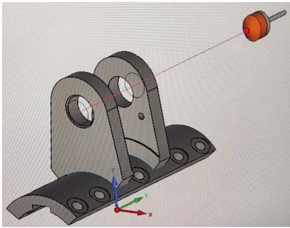
Slika 57. Simulacija bušenja provrta \phi 36 mm (lijevo) i proširivanje provrta \phi 44,6 mm (desno) [28]
