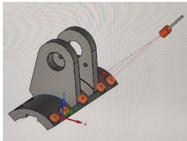
Slika 51. Simulacija izrada provrta (lijevo) te izrada upuštenja (desno) [28]
