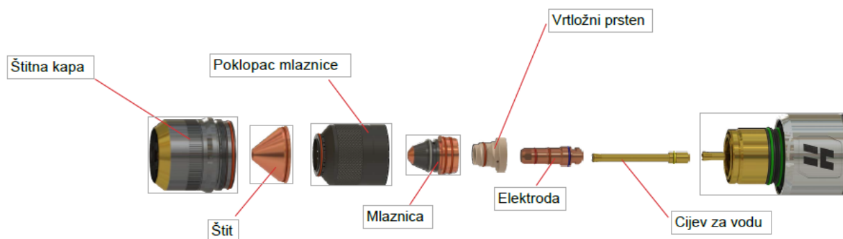
Slika 8. Prikaz dijelova pištolja za plazma rezanje [13]
