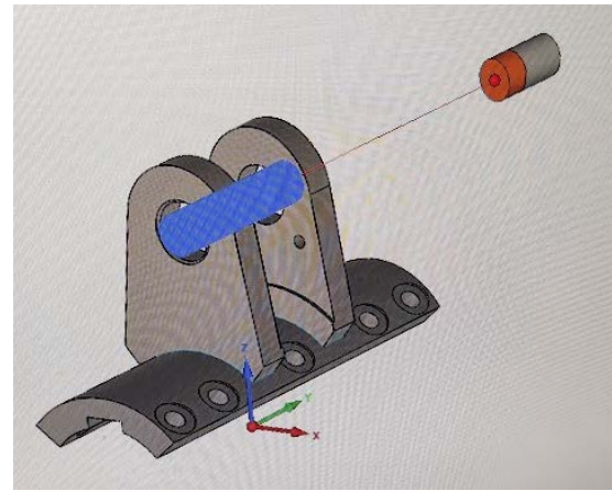
Slika 57. Simulacija bušenja provrta \phi 36 mm (lijevo) i proširivanje provrta \phi 44,6 mm (desno) [28]
