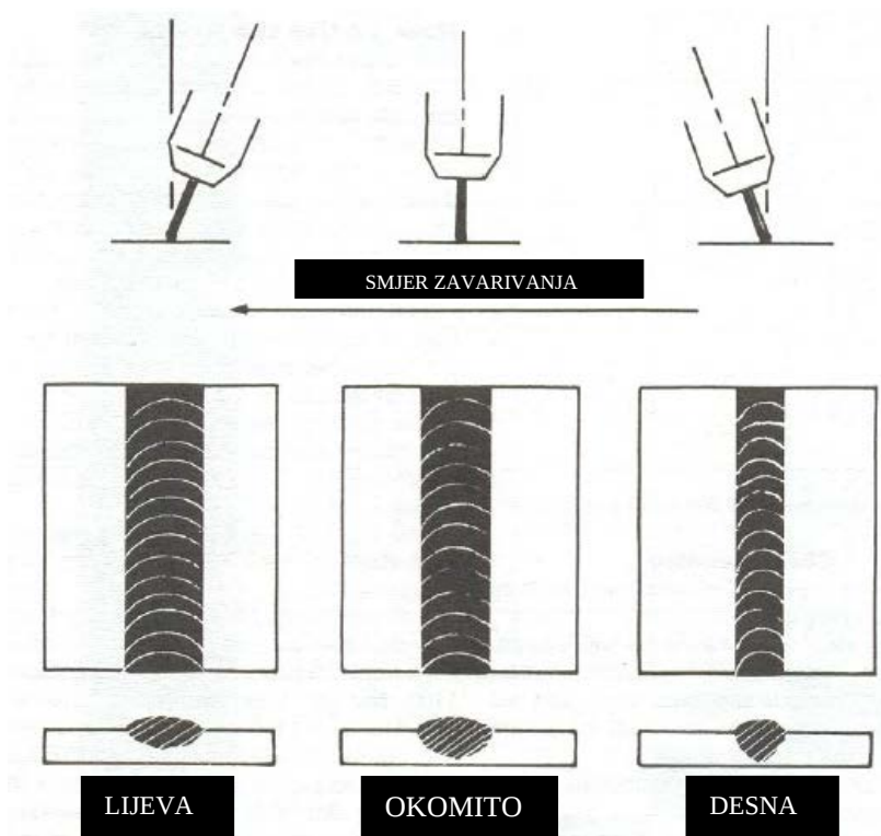
Slika 15. Tehnike zavarivanja [17]
