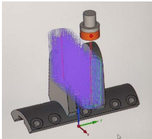
Slika 59. Simulacija finog glodanja postolja [28]
