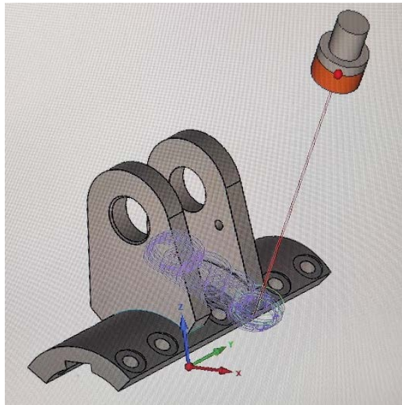
Slika 54. Simulacija glodanja na mjeru 64 mm s glodalom \phi 50 mm [28]
