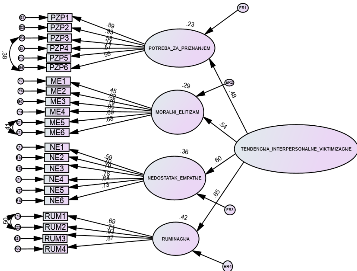
Slika 2. Konfirmatorna faktorska analiza drugog reda Skale tendencije interpersonalne viktimizacije, modificirani model
