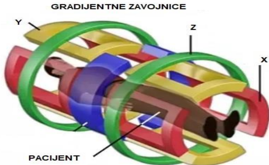
Slika 87. Shematski prikaz gradijentnih zavojnica
