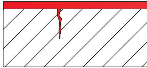
NANOŠENJE PENETRANTA
