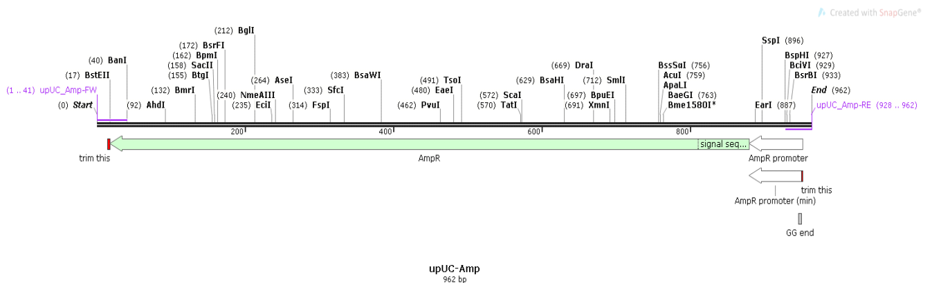
Slika 16. Amplificirani fragment amplicinske rezistencije iz pBackBoneBZ_ann (upUC-AmpR)
