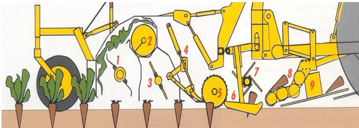
Slika 3.8. Uređaj za pripremu i vađenje šećerne repe: 1-sjekač lišća, 2-pužni transporter, 3-odstranjivač zaostaloga lišća, 4-sjekač glava, 5-taster za automatsko određivanje dubine vađenja, 6-vadilica, 7-čistač repe, 8-valjci za čišćenje, 9-sita
