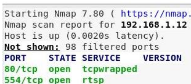
Slika 6-74 Zenmap DVC 192.168.1.12
