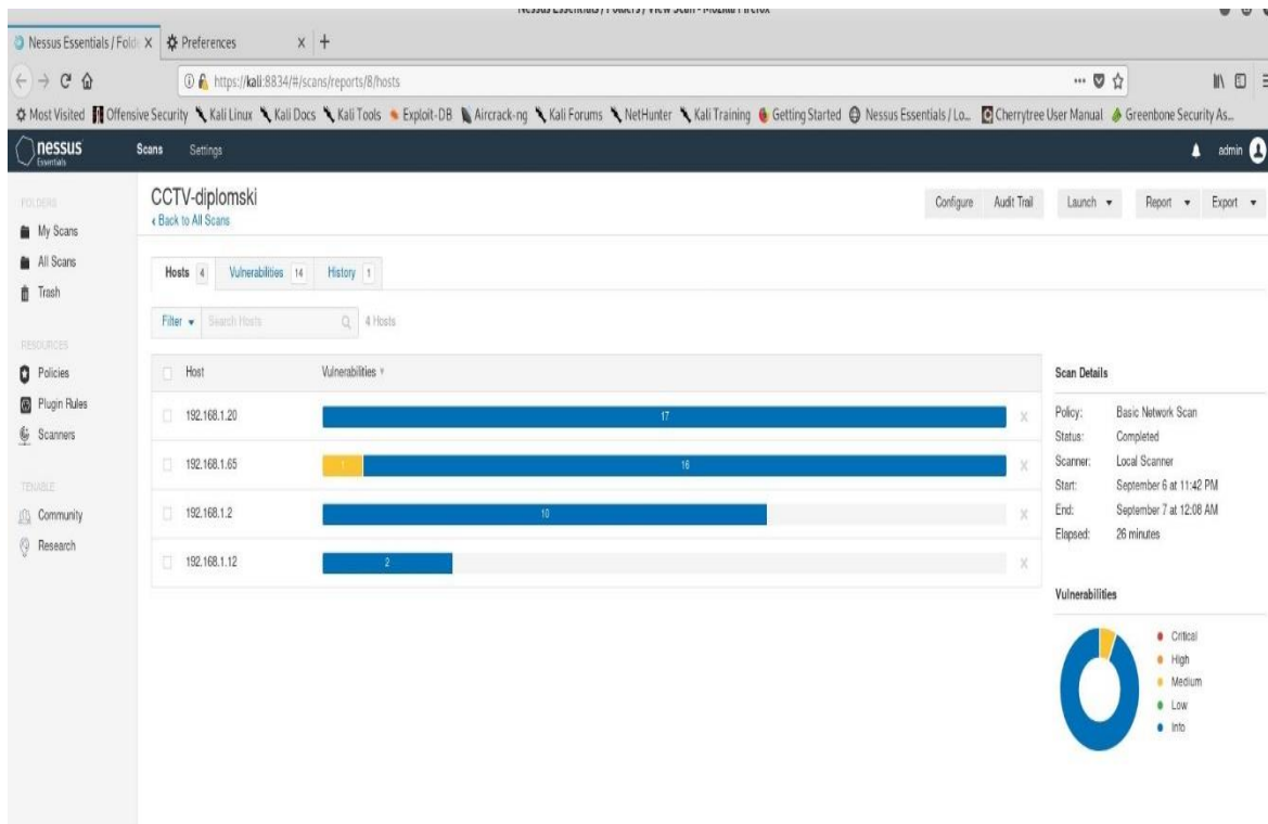
Slika 6-34 Nessus skeniranje
