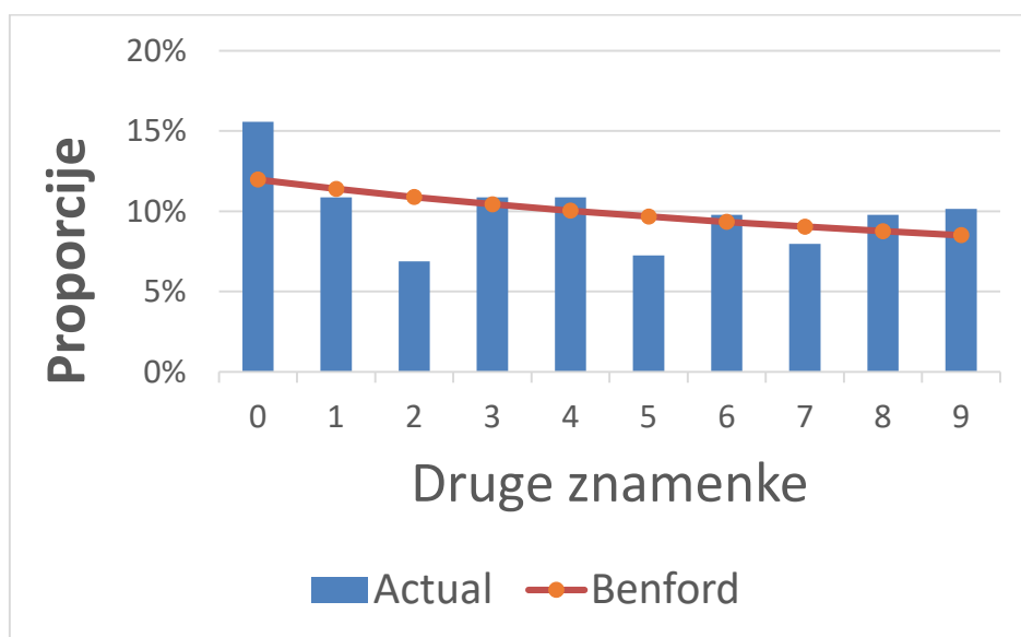
Grafikon 18: Stvarne i očekivane proporcije znamenki na drugoj brojevnoj poziciji dobiti poduzeća koja su revidirana od strane ostalih revizorskih društava
