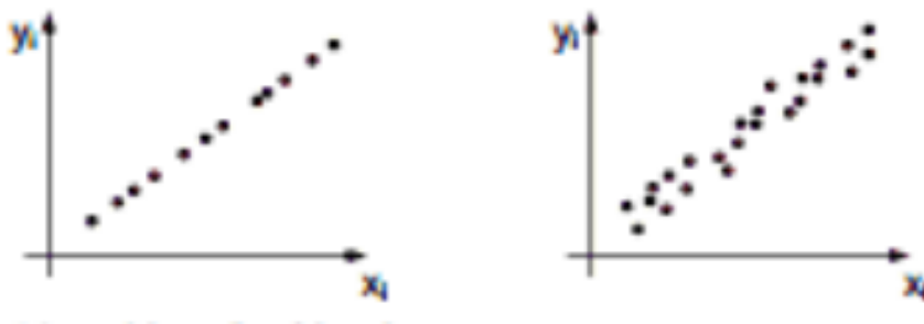
Slika 5.: Dijagram rasipanja
