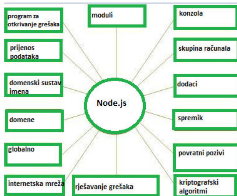
Slika 2.2. Node.js koncept [7]
