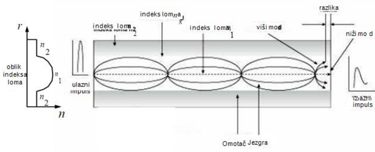
Slika 4.9 Prikaz višemodnog svjetlovoda sa gradijntnim indeksom loma [2].
