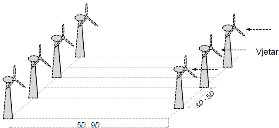
Sl. 4.13. Najpovoljnije rastojanje vjetroagregata [6]
