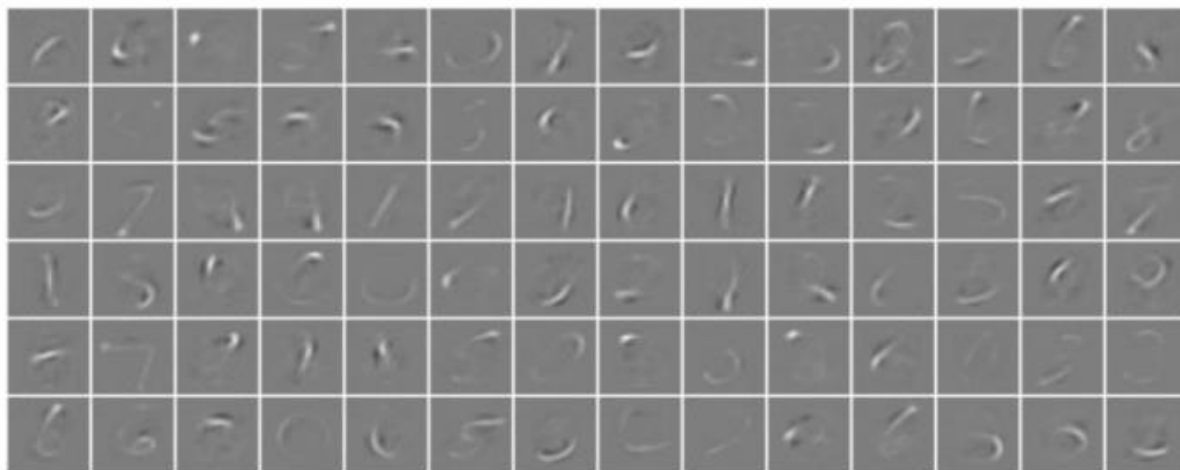
Sl. 3.4. Aktivacije preuzete iz prvog konvolucijskog sloja jednostavne duboke CNN mreže nakon obuke na MNIST bazi podataka, [22]
