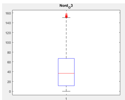
Sl. 4.3. Boxplot Nord|O 3 mjerenja
