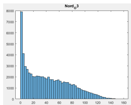
Sl. 4.4. Histogram Nord|O 3 mjerenja
