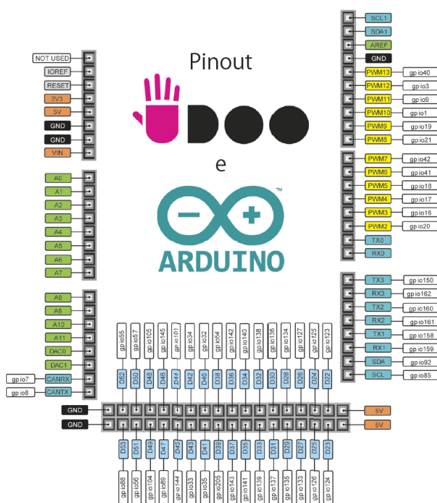
SI. 4.3. Raspored ulaza/izlaza Arduino Mega [7].
