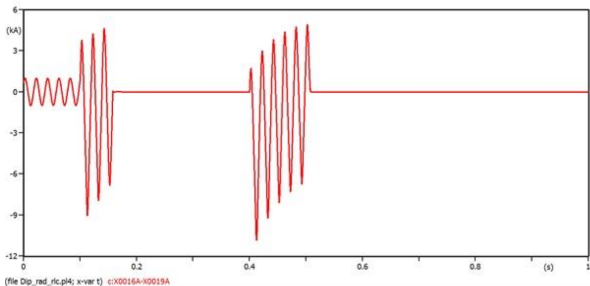
Sl. 5.8. Valni oblik struje faze A generatora pri jednofaznom kratkom spoju
