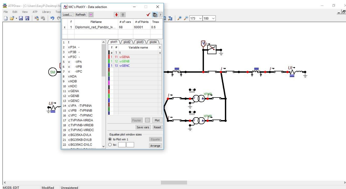
Sl.5.6.Prikaz grafičkih oblika napona i struja
