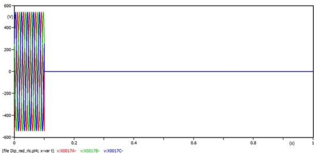
Sl. 5.31. Valni oblici napona pojedinih faza na mjestu kvara pri trofaznom kratkom spoju
