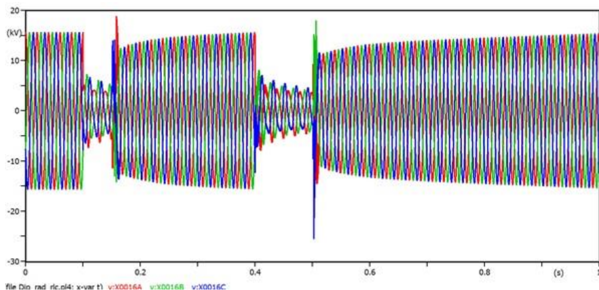
Sl. 5.20. Valni oblici napona pojedinih faza generatora pri trofaznom kratkom spoju
