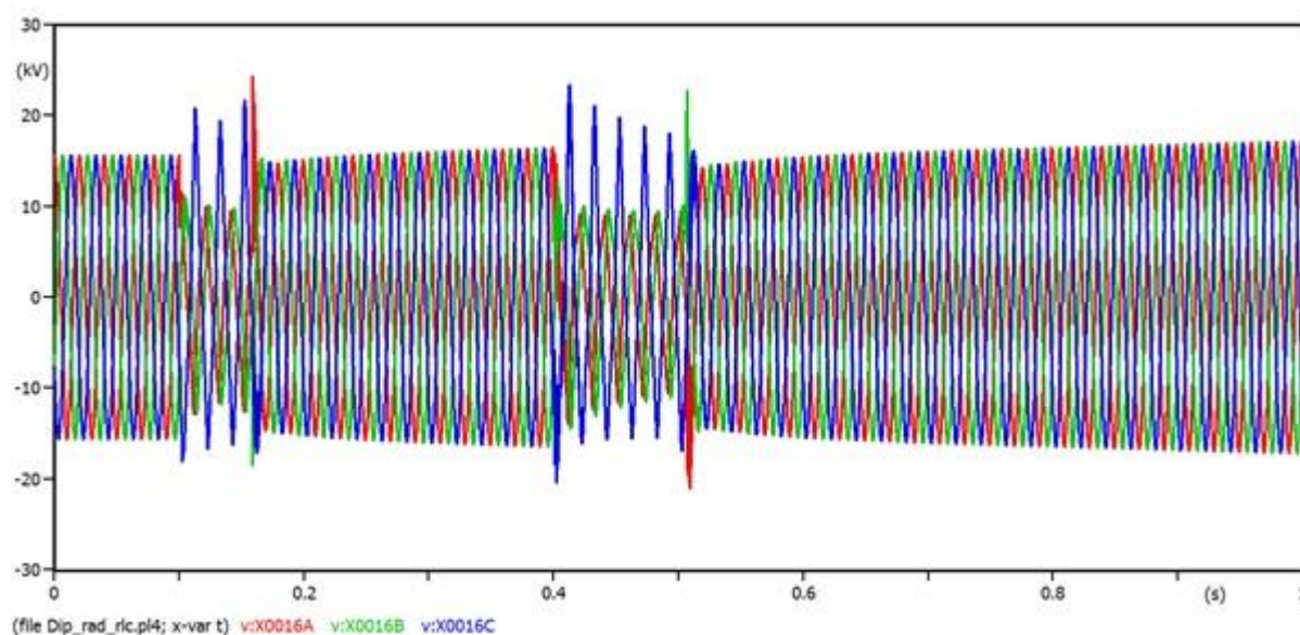
Sl. 5.16. Valni oblici napona pojedinih faza generatora pri jednofaznom kratkom spoju
