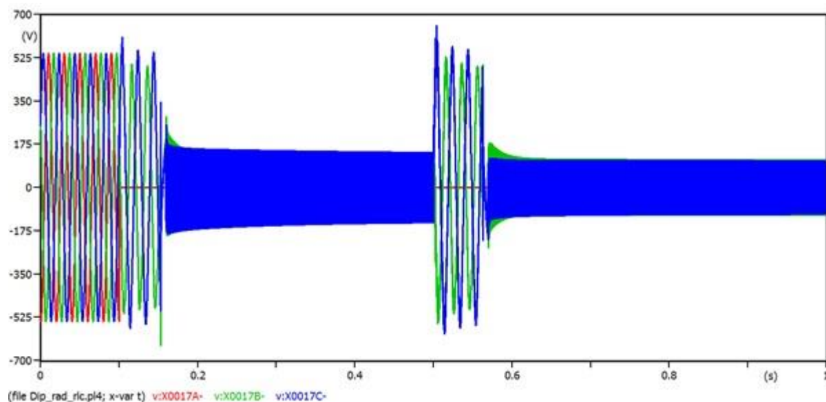
Sl. 5.27. Valni oblici napona pojedinih faza na mjestu kvara pri jednofaznom kratkom spoju
