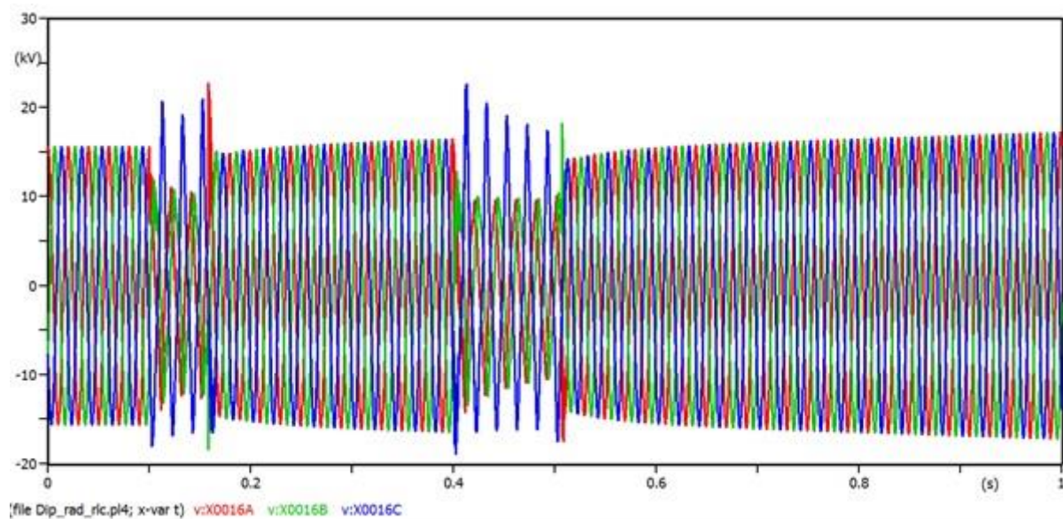
Sl. 5.7. Valni oblik napona pojedinih faza generatora pri jednofaznom kratkom spoju
