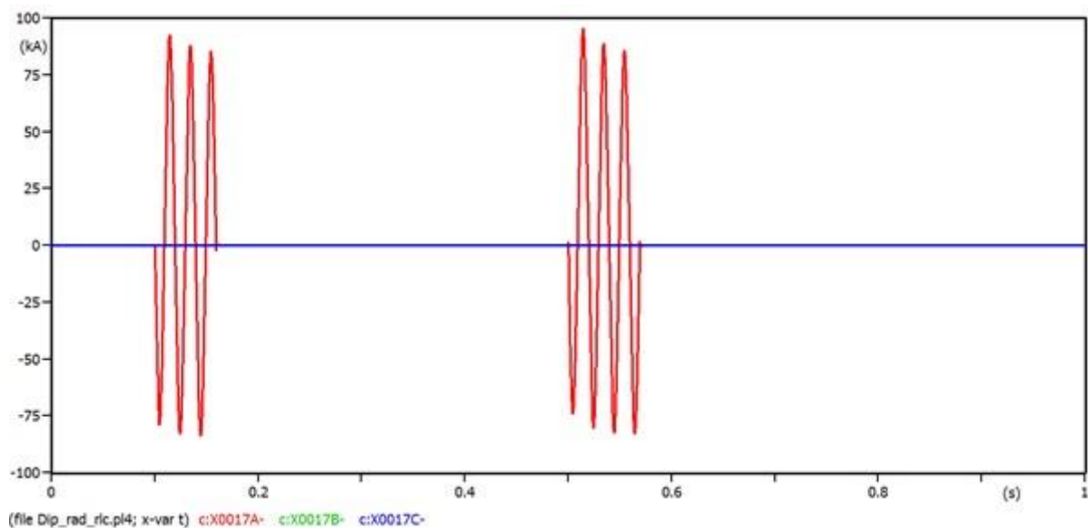
Sl. 5.26. Valni oblici struja pojedinih faza generatora pri jednofaznom kratkom spoju
