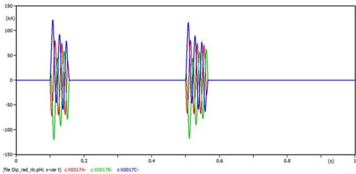
Sl. 5.30. Valni oblici struja pojedinih faza na mjestu kvara pri trofaznog kratkom spoju
