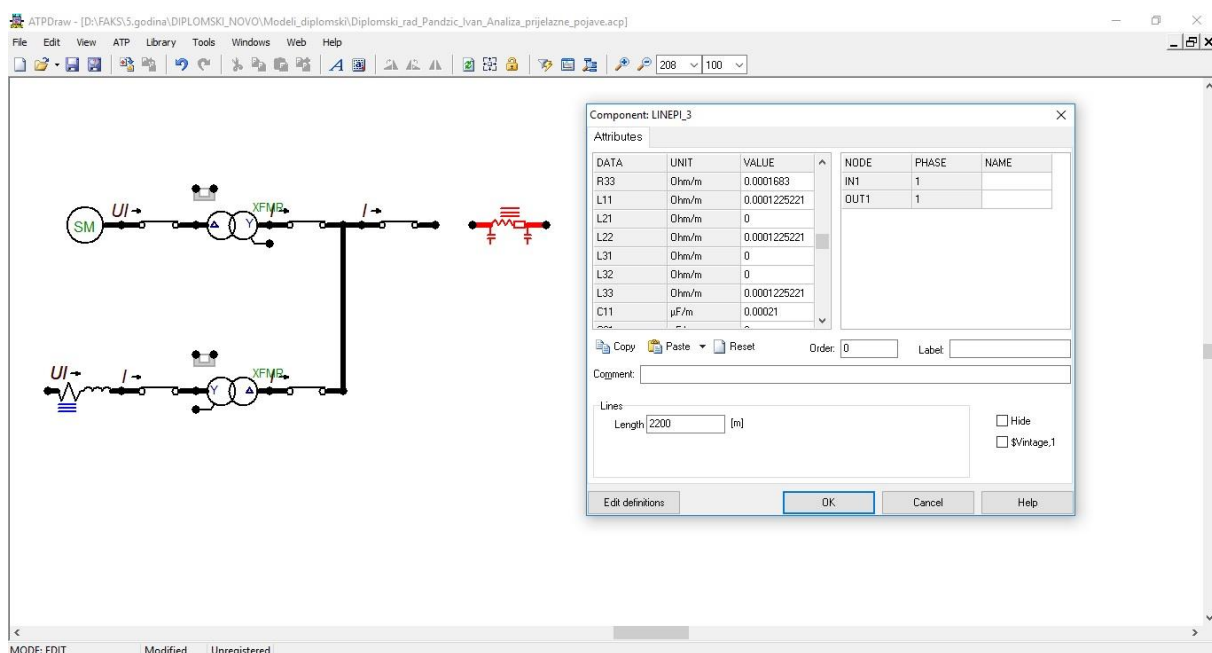
Sl. 4.11. Ulazni podaci kabla u ATPDraw-u
