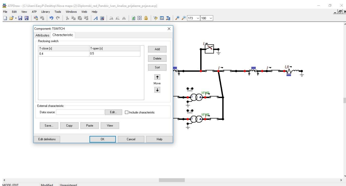
Sl. 5.3. Postavke automatskog ponovnog uklopa
