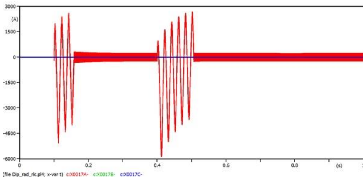
Sl. 5.9. Valni oblici struja pojedinih faza na mjestu kvara pri jednofaznom kratkom spoju
