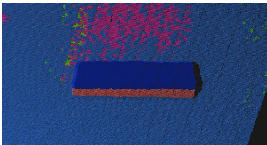
Slika 8.4.c Segmentirana slika
