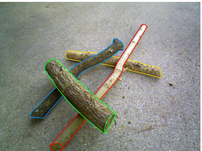
Slika 8.17.b Označeni bridovi
