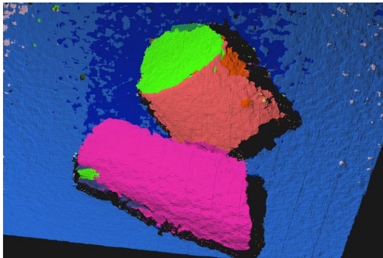
Slika 8.16.c Segmentirana slika
