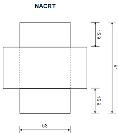
Slika 4.4 Nacrt transformatora
