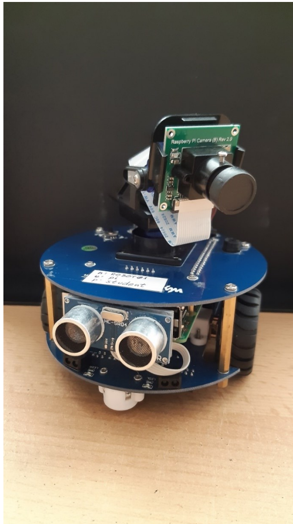
Slika 2.1 AlphaBot2 PI
