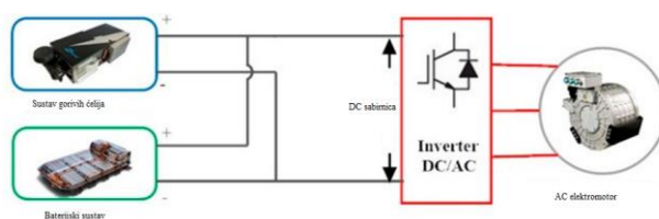
Slika 3. 12. Topologija 1
