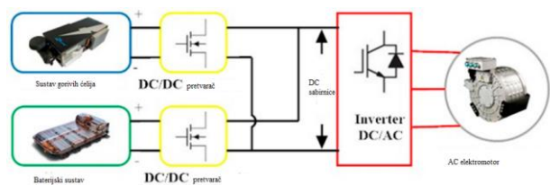
Slika 3. 15. Topologija 4
