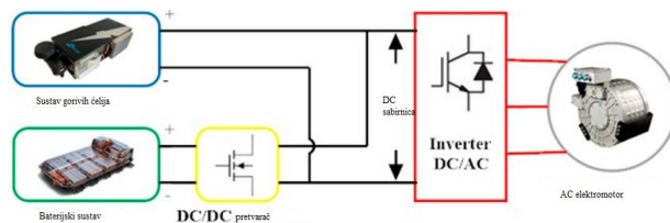
Slika 3. 14. Topologija 3
