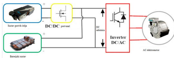
Slika 3. 13. Topologija 2
