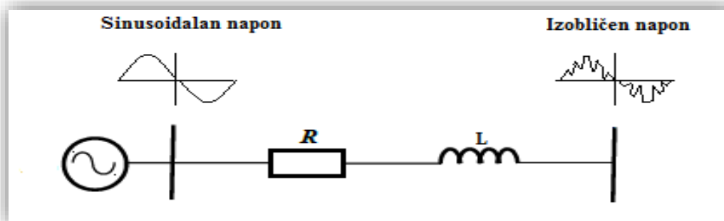
Slika 2.16. Izobličenje napona nelinearnim trošilom.
