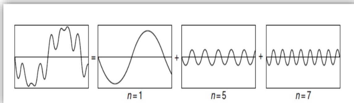
Slika 2.14. Dekompenzacija iskrivljenog valnog oblike u harmonijske komponente[2,str.189].
