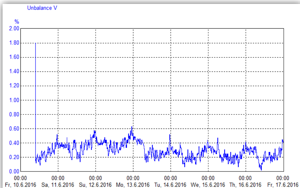
Slika 4.15. Nesimetrija napona u mjernom razdoblju.
