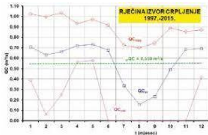
Slika 6. Crpljenje vode iz izvora Rječine [6].
