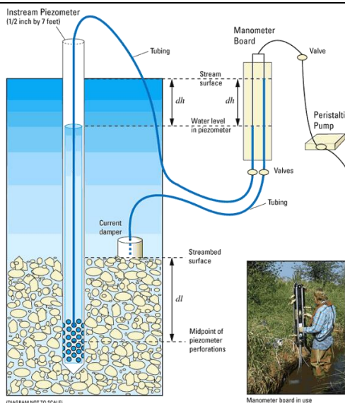
Slika 10. Piezometar- presjek [6].
