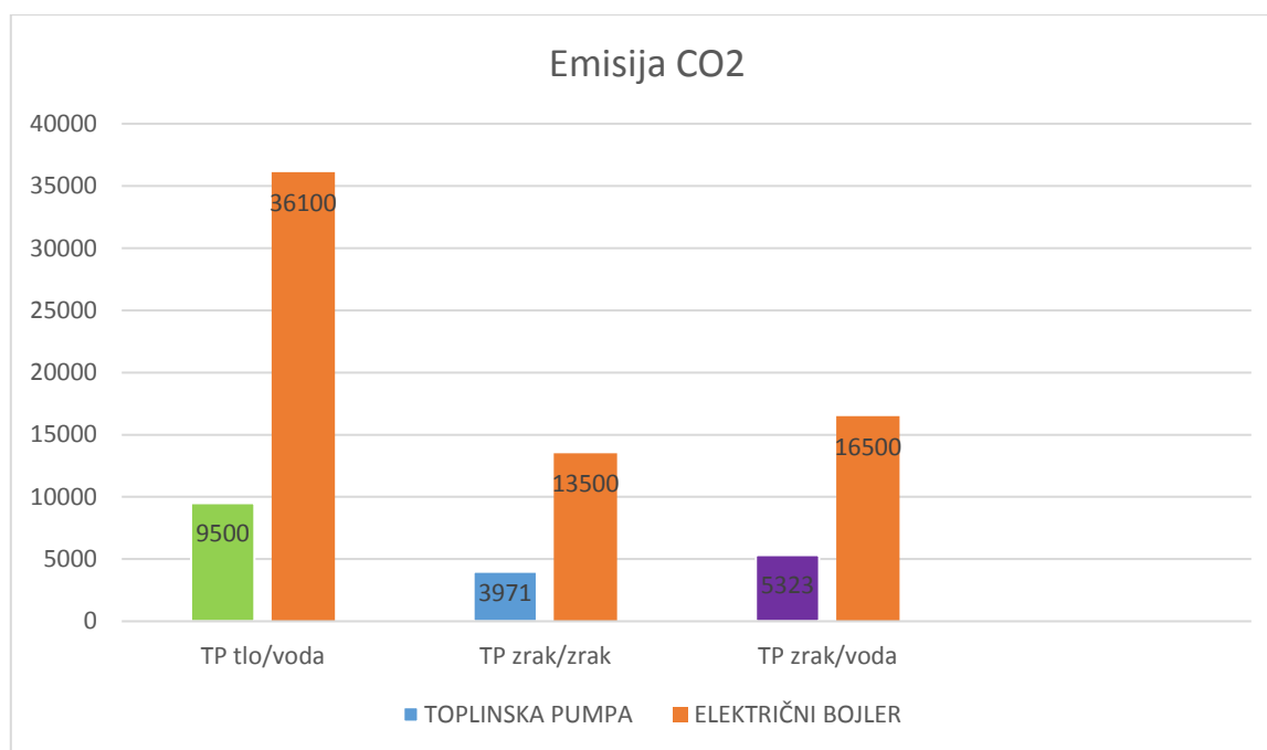
Dijagram 1: Količina emisije CO 2 u usporedbi sa električnim bojlerom [3]
