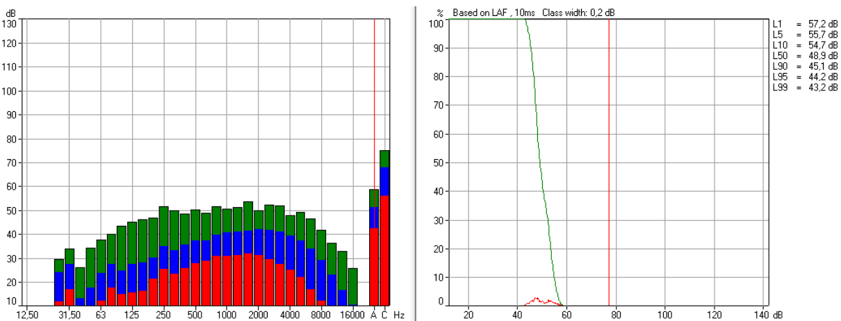
Slika 38. Frekvencijski spektar buke na lokaciji 8 sa otvorenim prozorima (lijevo) uz kumulativnu razdiobu i karakteristične statističke veličine (desno)
