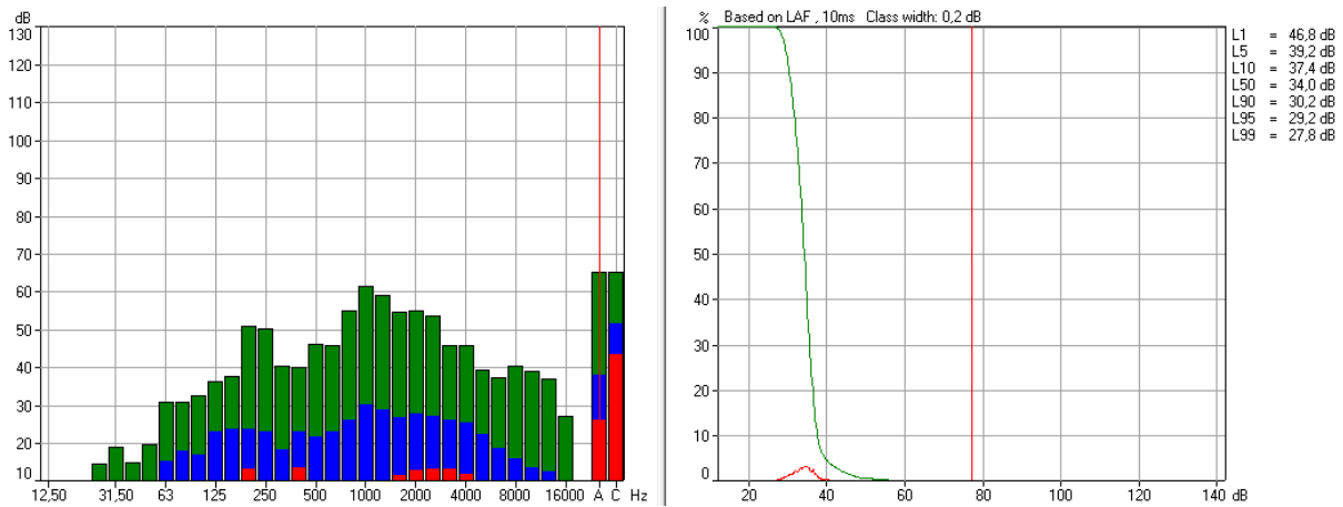
Slika 37. Frekvencijski spektar buke na lokaciji 8 sa zatvorenim prozorima (lijevo) uz kumulativnu razdiobu i karakteristične statističke veličine (desno)
