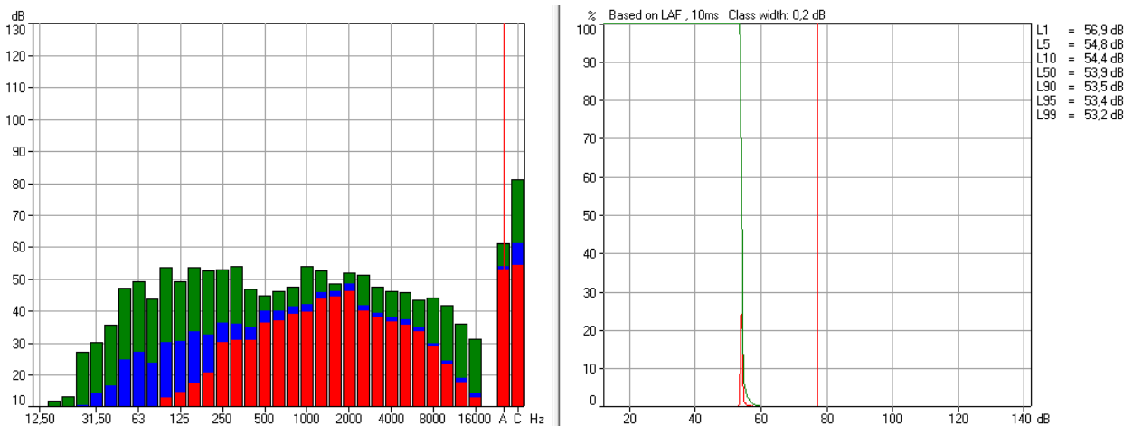
Slika 46. Frekvencijski spektar buke na lokaciji 7 sa otvorenim vratima i zatvorenim prozorima (lijevo) uz kumulativnu razdiobu i karakteristične statističke veličine (desno)
