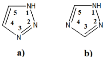
Slika 10. Izomeri triazola: a) 1,2,3-triazol i b) 1,2,4-triazol
