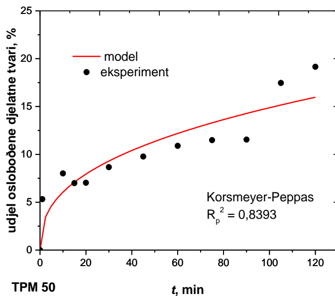
Slika 5.30. Testiranje primjenjivosti Korsmeyer-Peppas modela u opisu profila oslobađanja lurasidon-hidroklorida iz tableta TPM 50.
