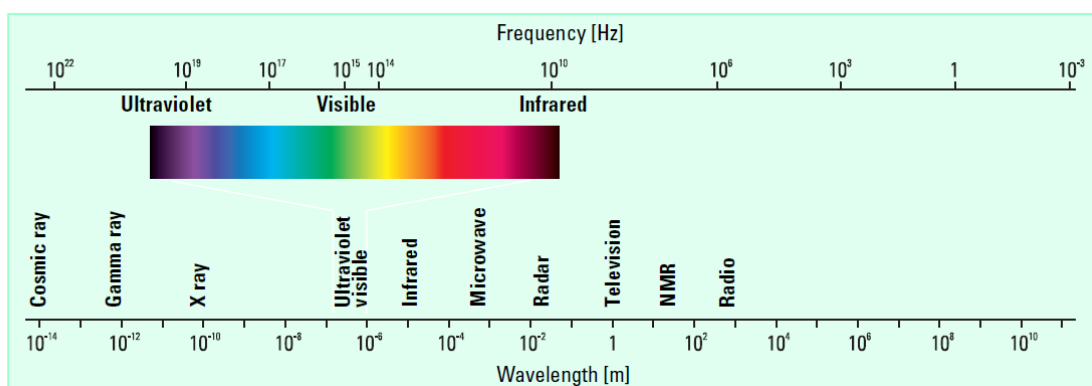
Slika 13. Elektromagnetski spektar
