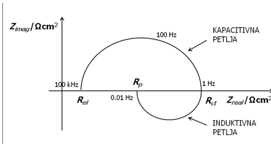
Slika 12. Nyquistov dijagram [1]
