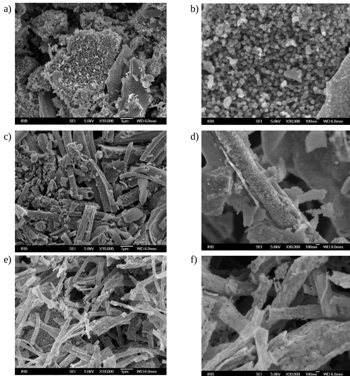
Slika 4.5. FE-SEM snimke termički obrađених vlakana dobivenih elektroispredanjem na udaljenosti 5 cm (a i b), 10 cm (c i d) i 15 cm (e i f).
