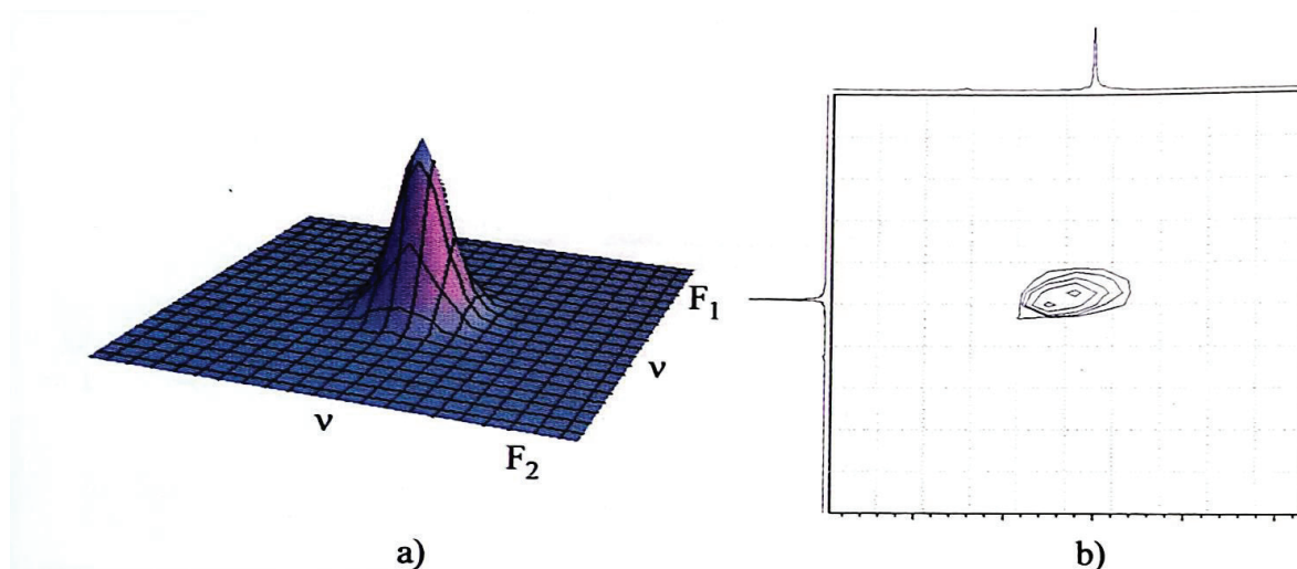
Slika 11: Shematski prikaz signala u dvodimenzijском спекtru NMR: a) trodimenzijski prikaz, b) konturni prikaz
