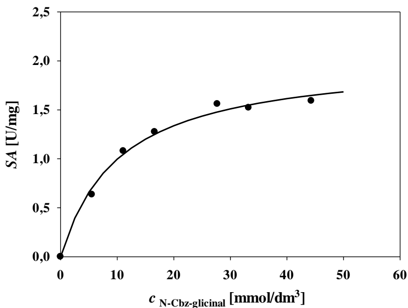
Slika 5.2. Utjecaj koncentracije N-Cbz-glicinala na specifičnu aktivnost enzima u reakciji aldolne adicije ( \gamma_{FSA} = 0,25 \text{ mg/cm}^3 , c_{N-Cbz-glicinala} = 0-45 \text{ mmol/dm}^3 , c_{DHA} = 100 \text{ mmol/dm}^3 , 10 % (v/v) acetonitrila, 50 \text{ mmol/dm}^3 TEA-HCl pufer pH 8,0, 25^\circ\text{C} , V_{reaktor} = 0,5 \text{ cm}^3 ).
