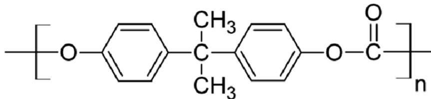
Slika 8. Strukturni prikaz polikarbonata 19
