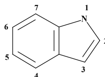
Fig. 4. Indole.
