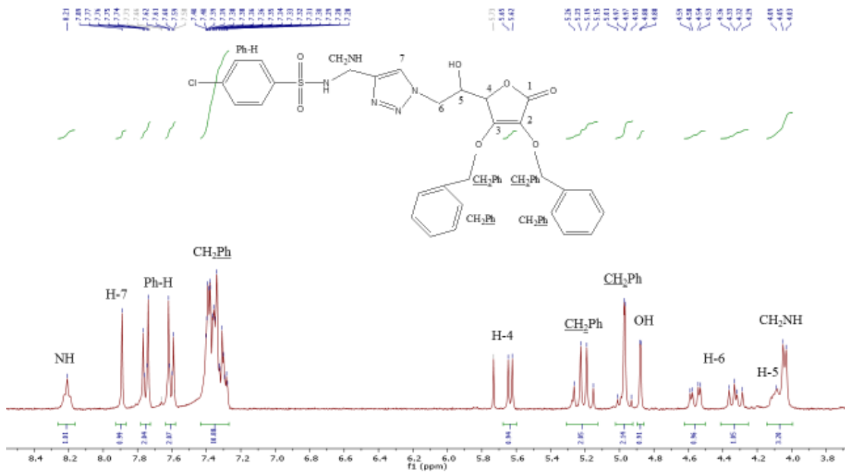
Slika 28. Spektar 1 H-NMR spoja 22
