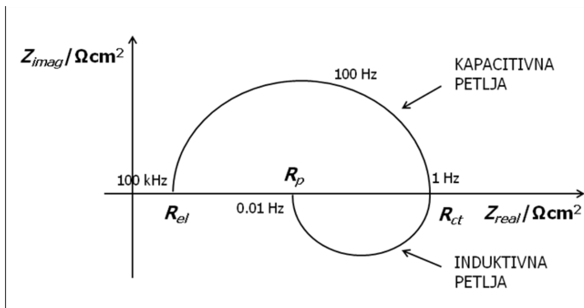
Slika 12. Nyquistov dijagram [1]
