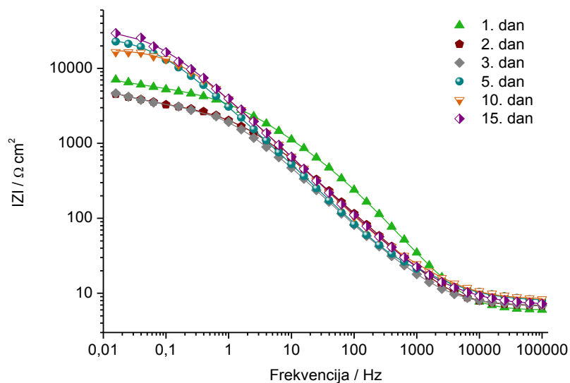
Slika 21. a) i b) Bodeov prikaz impedancijskih krivulja za uzorak tretiran stearinskom kiselinom, c(\text{SK})=10^{-3}\text{M} u ovisnosti o vremenu.
