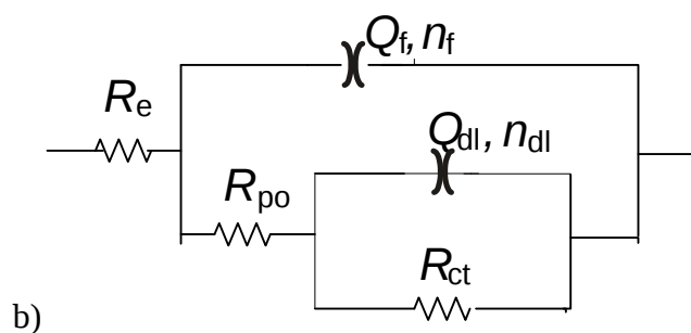
Slika 19. Električni ekvivalentni krugovi korišteni za modeliranje eksperimentalnih podataka
