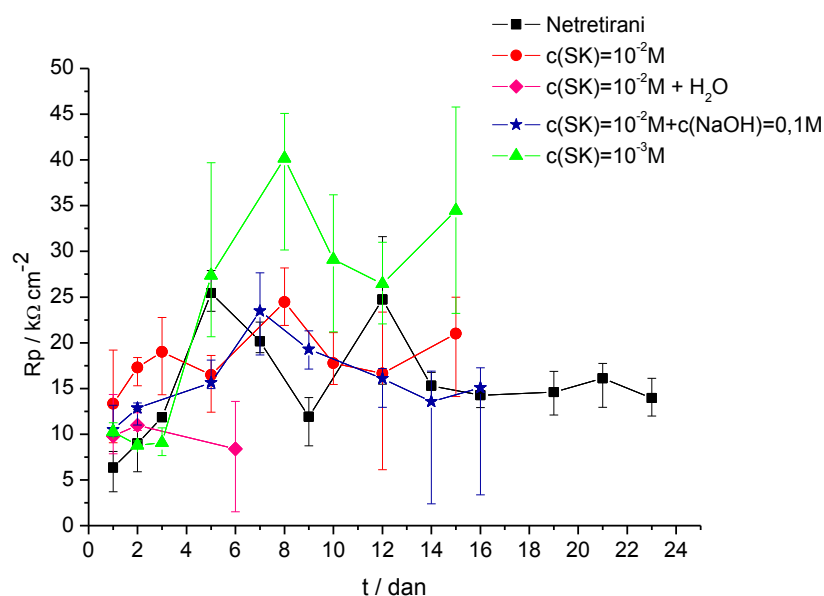
Slika 16. Ovisnost polarizacijskih otpora za netretirani i tretirane uzorke o vremenu.
