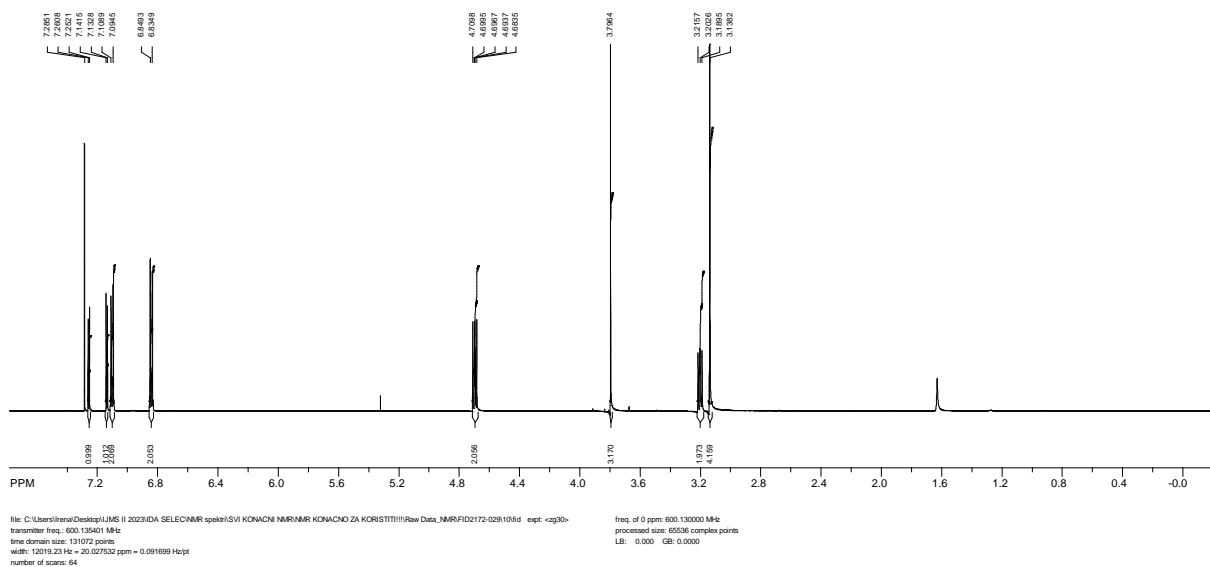
Slika 29. ^1\text{H} NMR ( \text{CDCl}_3 ) spektar tienobenzotriazola 5 , nearomatskog para spoja 12 .
