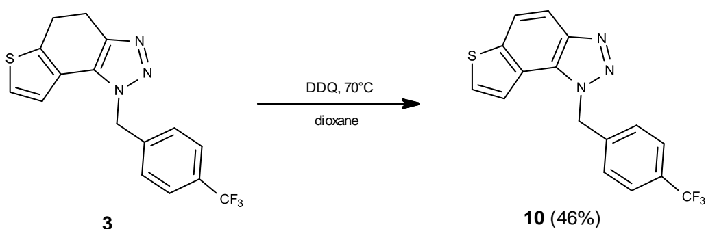
Shema 14. Sintaza 1-(4-(trifluorometil)benzil)-1 H -tieno[3',2':3,4]benzo[1,2- d ][1,2,3]triazola ( 10 ).
