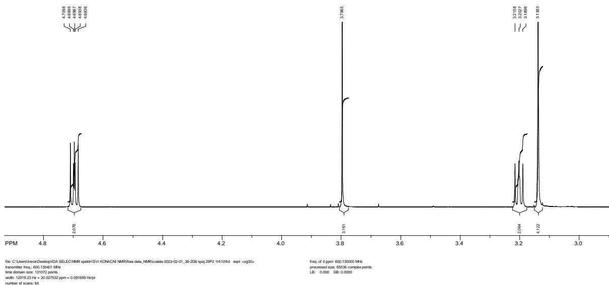
Slika 30. Alifatski dio ^1\text{H} NMR ( \text{CDCl}_3 ) spektra tienobenzotriazola 5 .
