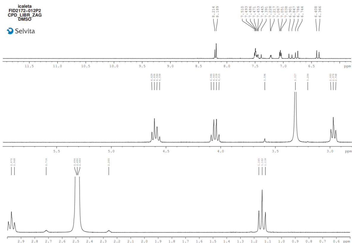
Slika 17. ^1\text{H} NMR ( \text{CDCl}_3 ) spektar početnog tieno-triazolostilbena.
