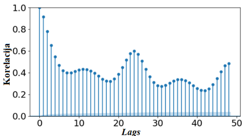
Slika 4.6. Prikaz autokorelacije koncentracije \text{NO}_2
