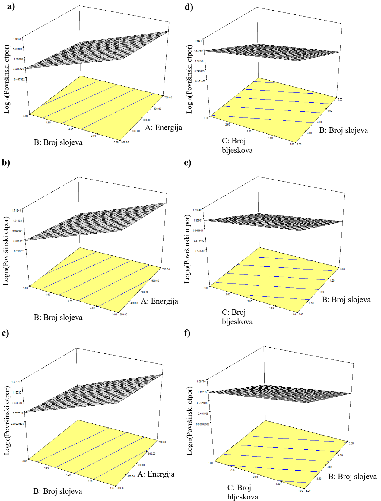
Slika 4.48. 3D grafički prikaz ovisnosti logaritma površinskog otpora o energiji i broju slojeva za: a) 1, b) 2 i c) 3 bljeska i ovisnost logaritma površinskog otpora o broju slojeva i broju bljeskova za energije od: d) 300 J, e) 500 J i f) 700 J.
