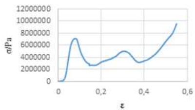
Slika B7. Krivulja naprezanje – deformacija za uzorak P u drugom tjednu razgradnje.
