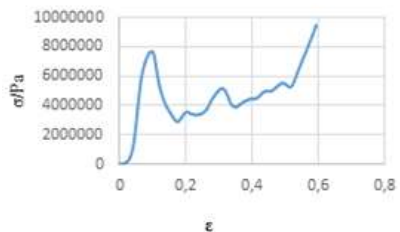
Krivulja naprezanje – deformacija za uzorak 2P5
