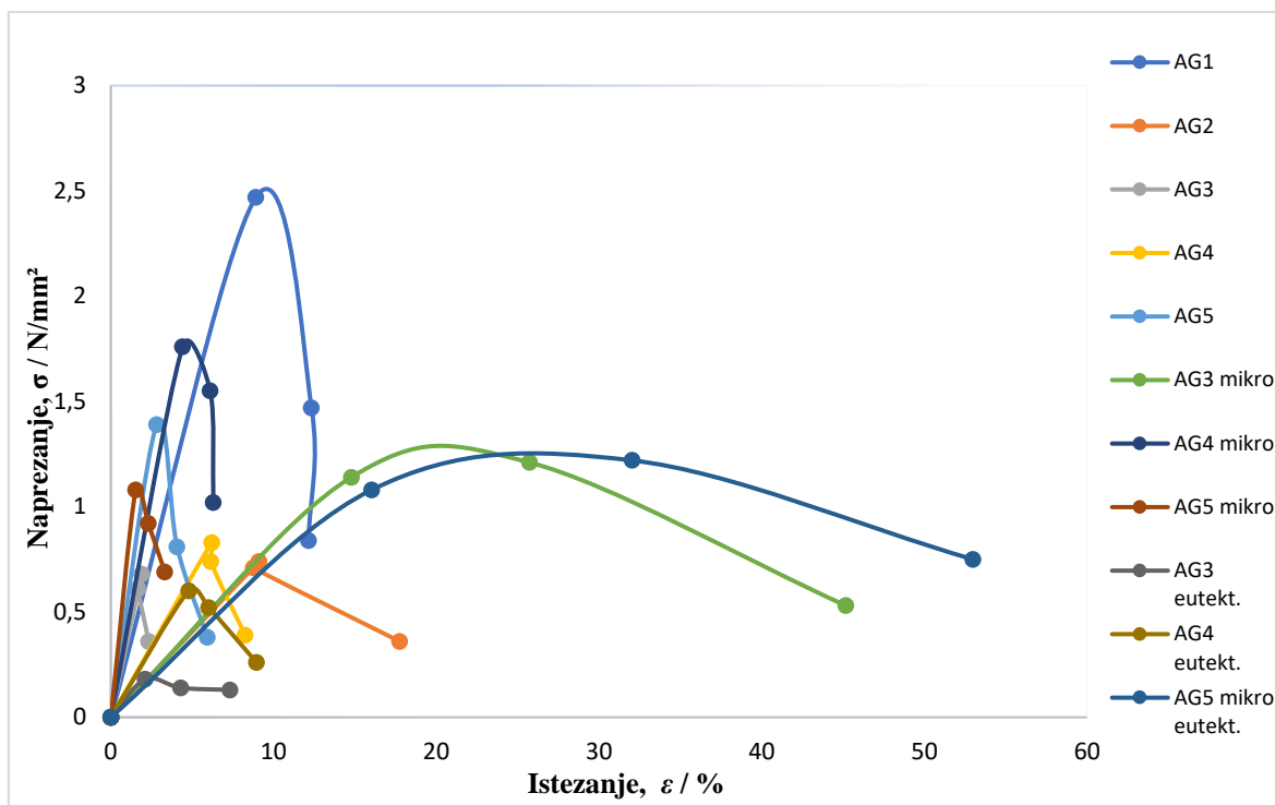
Slika 20. Grafički prikaz ovisnosti naprezanje/deformacija TPS/celuloza mješavina.
