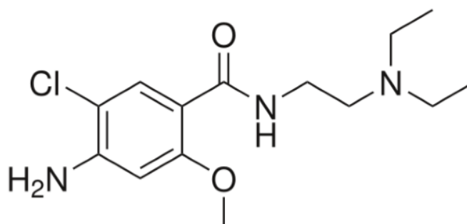
Slika 13. Struktura metoklopramida [56]
